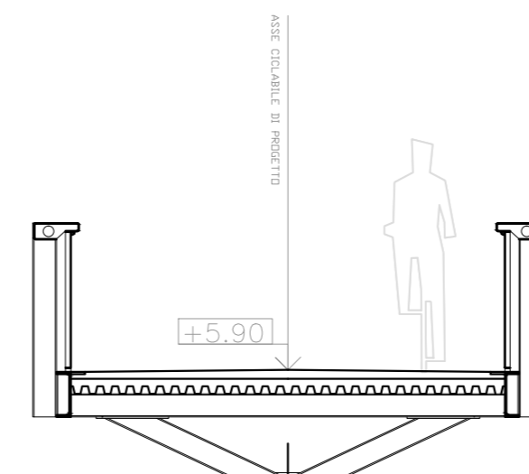
Sezione tipo profilo 1 scala 1:50
