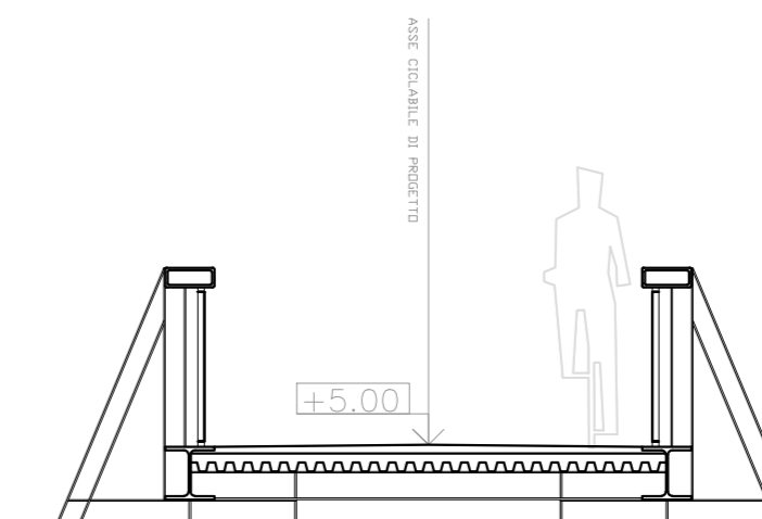
Sezione tipo profilo 2 scala 1:50
