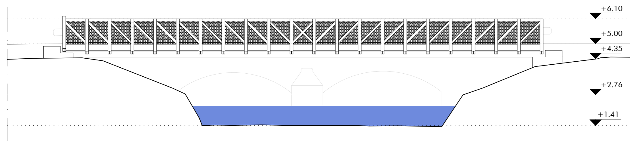
Profilo 2 scala 1:100
